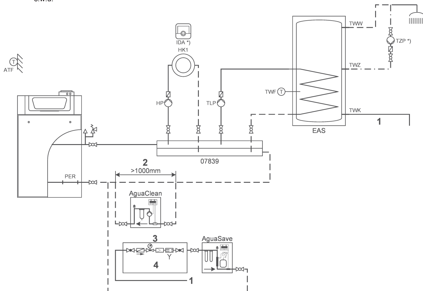
Rys.7 Kocioł BGB z podgrzewaczem c.w.u.: obieg c.o. z regulatorem pokojowym i z regulacją temperatury w podgrzewaczu c.w.u.
