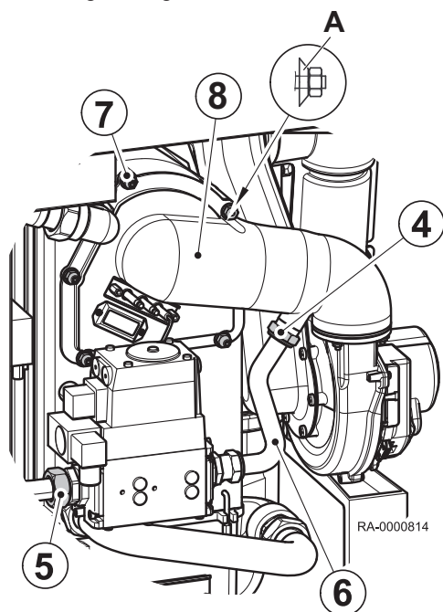
Rys.33 Wymontowywanie palnika gazowego
