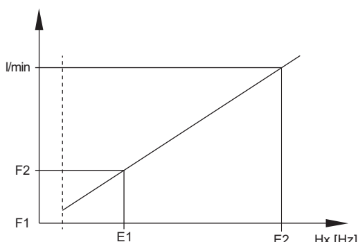
Rys.29 Przykład dwóch różnych charakterystyk czujnika
