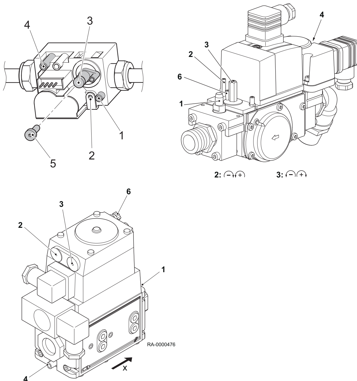
Rys.15 Zawór gazu
