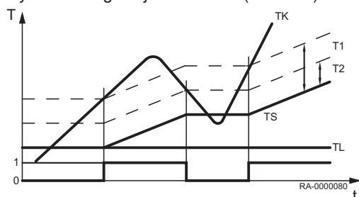
Rys.26 Regulacja ładowania (schemat)
