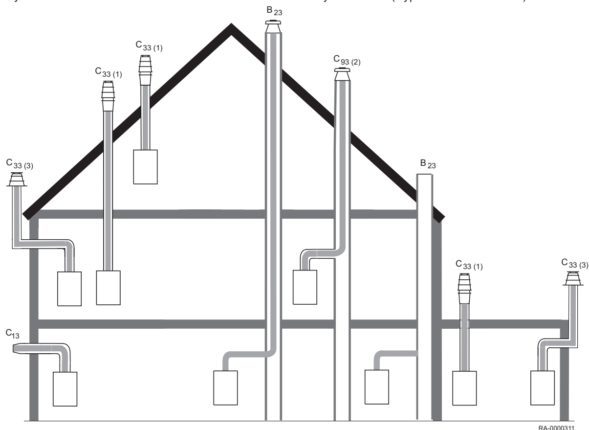
Rys.10 Możliwości zamontowania kotła z zastosowaniem systemu KAS (wyposażenie dodatkowe)
