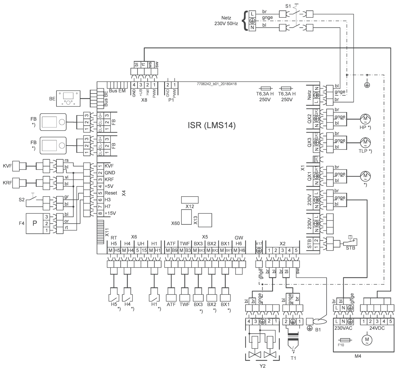
Rys.2 Schemat połączeń elektrycznych BGB 50
