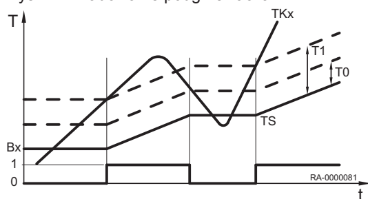
Rys.27 Ładowanie podgrzewacza
