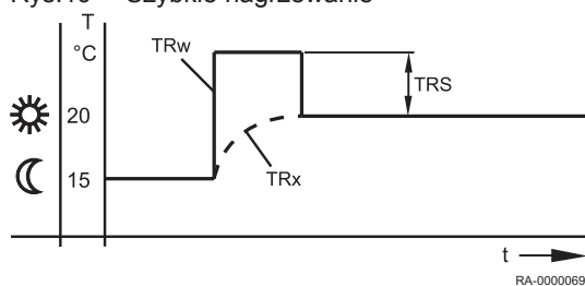
Rys.19 Szybkie nagrzewanie
