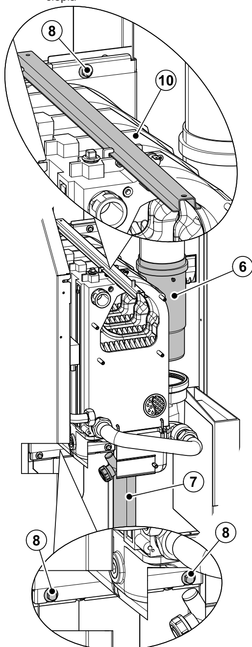
Rys.34 Wymontowywanie wymiennika ciepła
