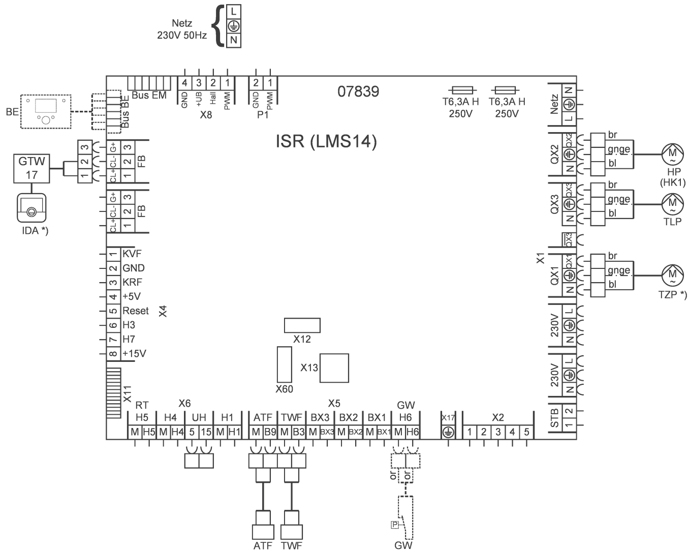
Rys.8 Schemat połączeń elektrycznych
