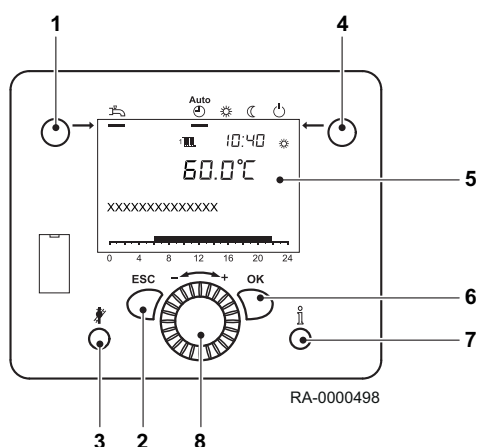
Rys.32 Elementy obsługowe
