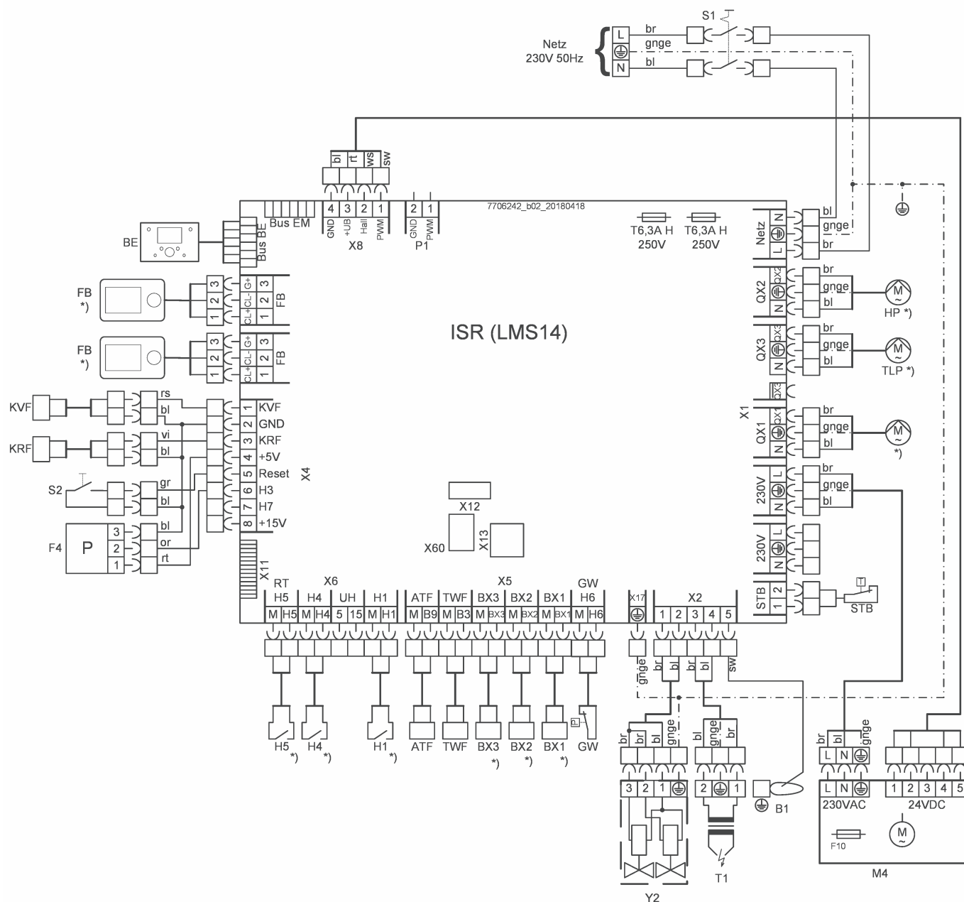
Rys.3 Schemat połączeń elektrycznych BGB 70 - 110
