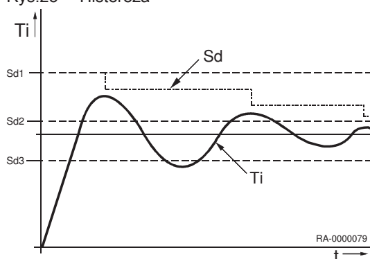
Rys.25 Histereza
