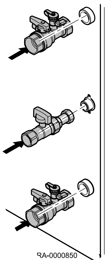
Rys.9 Montaż zaworów odcinających
