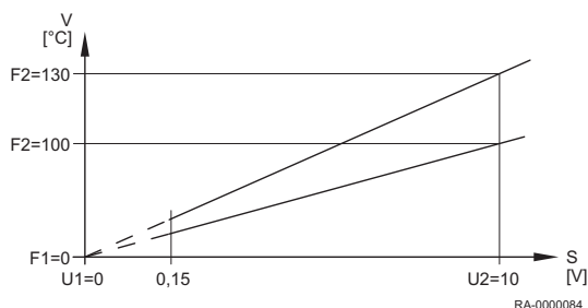
Rys.30 Przykład zapotrzebowania na ciepło 10 V
