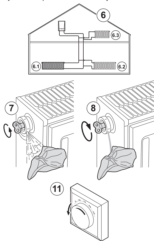
Rys.22 Odpowietrzanie instalacji
