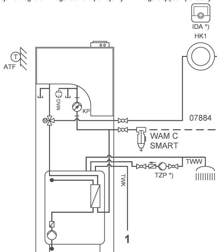
Rys.10 Przykładowa instalacja: obieg c.o. z regulatorem pokojowym i z regulacją temperatury w podgrzewaczu c.w.u.
