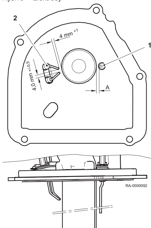
Rys.45 Elektrody
