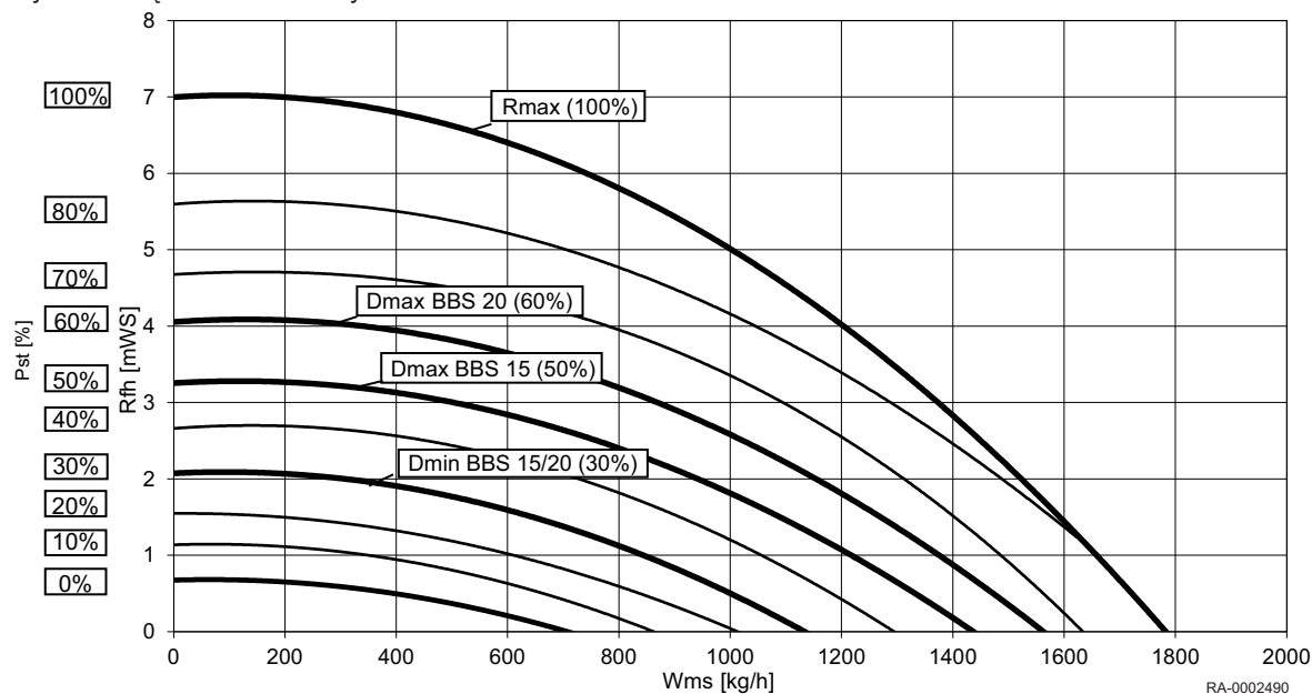
Rys.1 Łączne ciśnienie dynamiczne dla kotła BBS EVO 15 - 20
