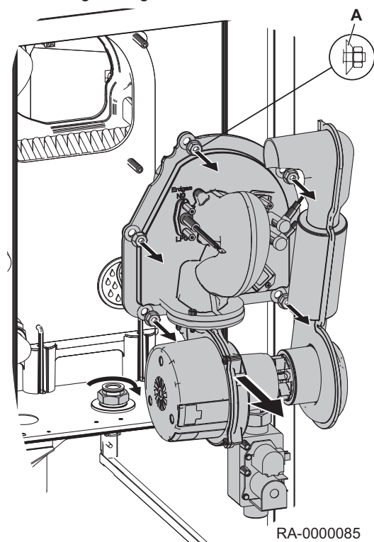
Rys.47 Wymontowywanie palnika gazowego
