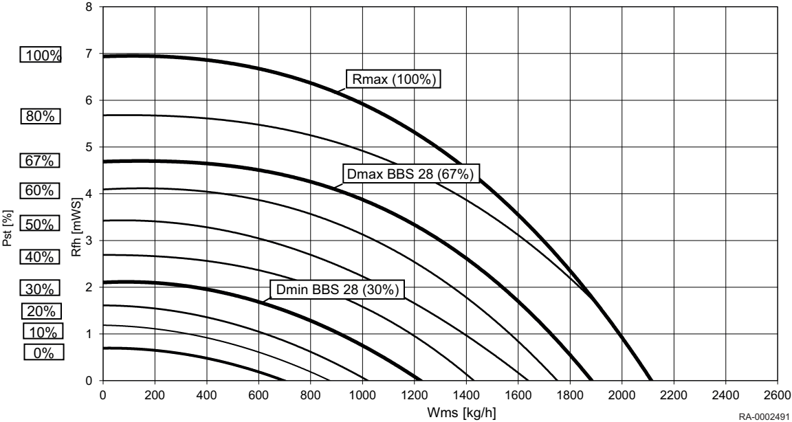
Rys.2 Łączne ciśnienie dynamiczne dla kotła BBS EVO 28
