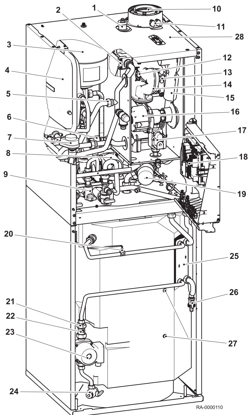
Rys.5 Widok kotła BBS EVO (bez przedniej ścianki i osłony regulatora)
