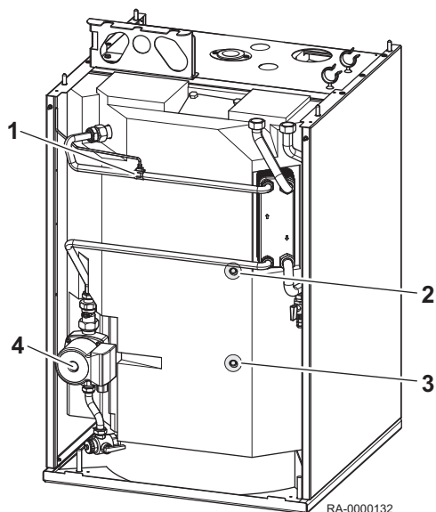
Rys.27 Warstwowy podgrzewacz c.w.u. (SSP)
