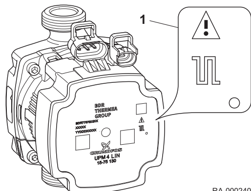
Rys.30 Wyświetlacz stanu pompa obiegowa c.o. UPM4
