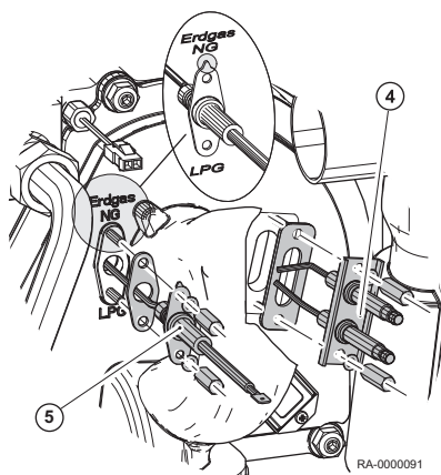
Rys.46 Wymontowywanie elektrody zapłonowej i jonizacyjnej
