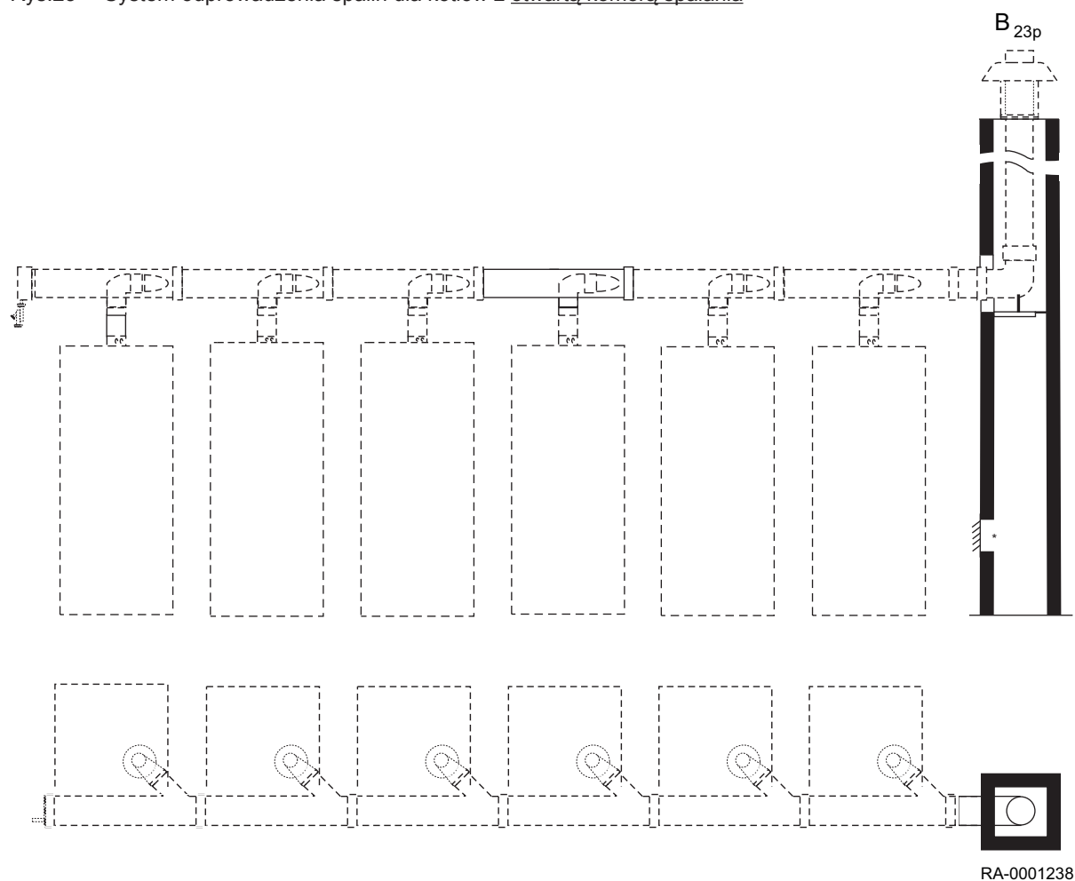
Rys.23 System odprowadzenia spalin dla kotłów z otwartą komorą spalania
