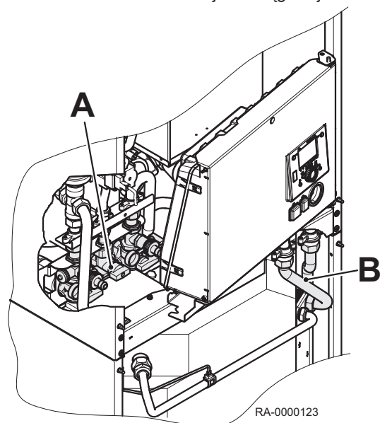
Rys.17 Podłączenie kotła i podgrzewacza c.w.u. do instalacji rurociągowej
