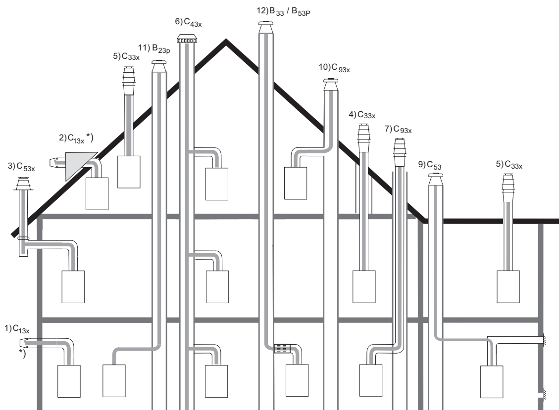
Rys.19 Możliwości zamontowania kotła z zastosowaniem systemu KAS (wyposażenie dodatkowe)
