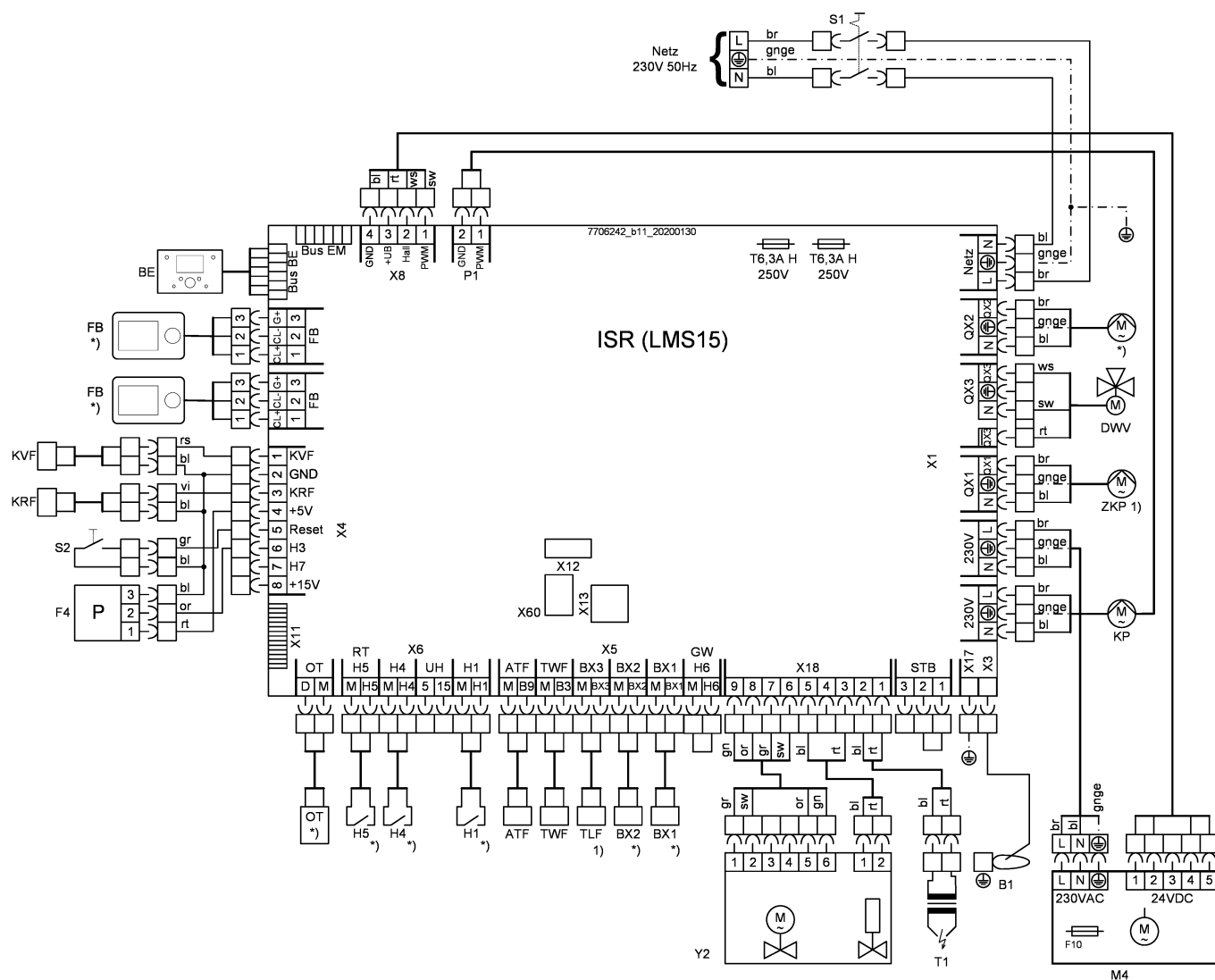
Rys.4 Schemat połączeń elektrycznych BBS EVO 15 - 28
