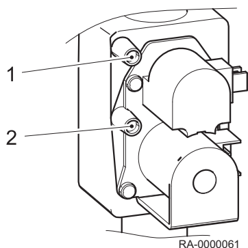
Rys.29 Zawór gazu BBS EVO
