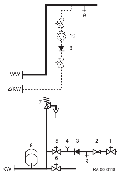
Rys.12 Podłączenie wody zimnej zgodnie z obowiązującymi normami i przepisami
