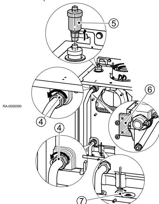
Rys.48 Wymontowywanie wymiennika ciepła
