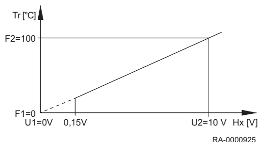
Rys.42 Wartość_napięcia/Wartość_funkcji
