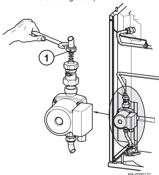
Rys.18 Zmiana kryzy wylotu gorącej wody (wyłącznie w przypadku zasobnika warstwowego SSP)
