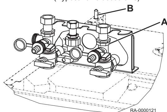
Rys.15 Podłączenie hydrauliczne
