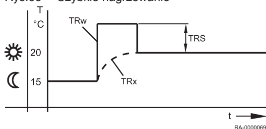
Rys.35 Szybkie nagrzewanie
