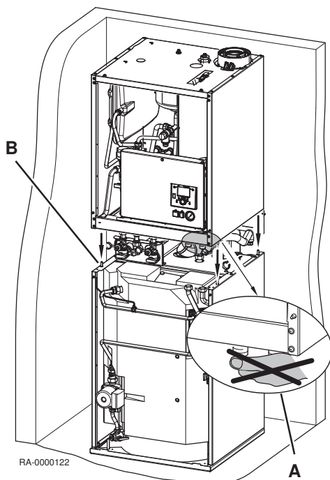
Rys.16 Montaż kotła
