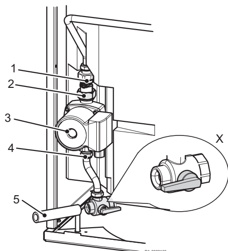
Rys.49 Wymontowywanie pompy ładującej podgrzewacz c.w.u.
