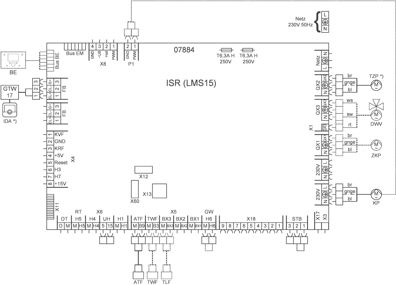
Rys.11 Schemat połączeń elektrycznych
