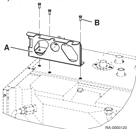
Rys.14 Mocowanie zestawu odcinającego AEH (wyposażenie dodatkowe)
