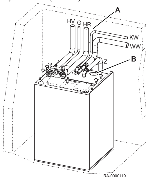
Rys.15 Podłączenie hydrauliczne
