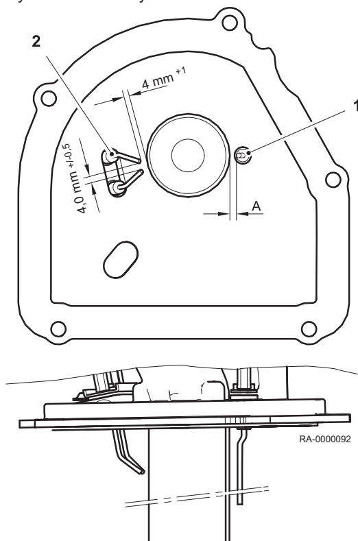
Rys.62 Elektrody
