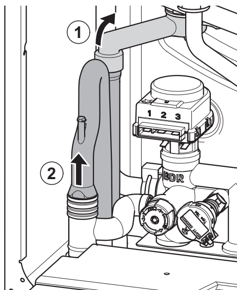
Rys.61 Wymontowywanie syfonu
