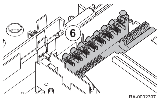
Rys.27 Płytki obwodów drukowanych, CB
