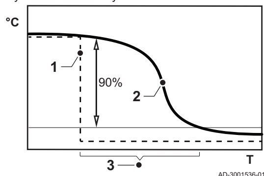
Rys.51 Bezwł budynku
