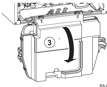
Rys.60 Wychylanie regulatora kotła całkowicie do dołu.
