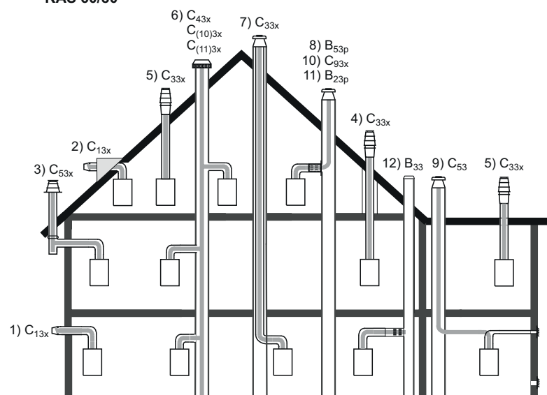
Rys.19 Odprowadzanie spalin w przypadku zastosowania systemu KAS (wyposażenie dodatkowe)
