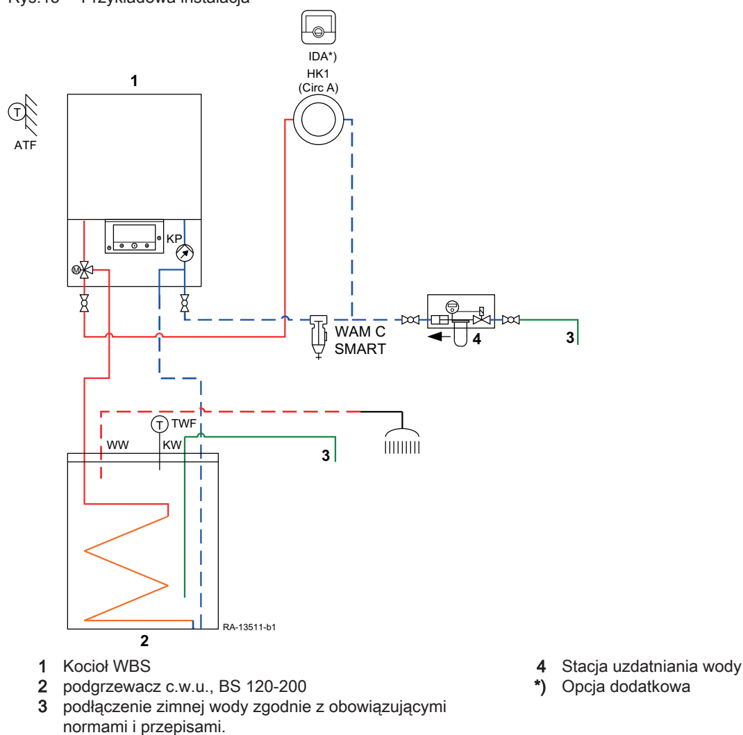
Rys.15 Przykładowa instalacja
