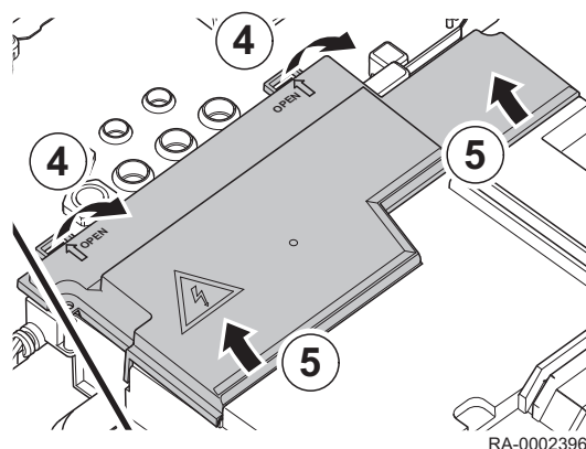
Rys.27 Płytki obwodów drukowanych, CB
