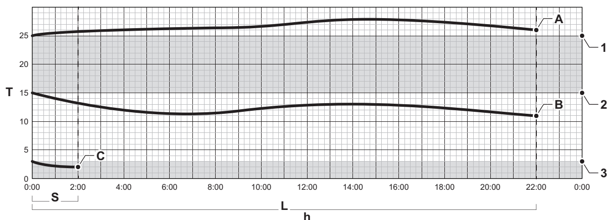
Rys.53 Przełączanie między latem i zimą
