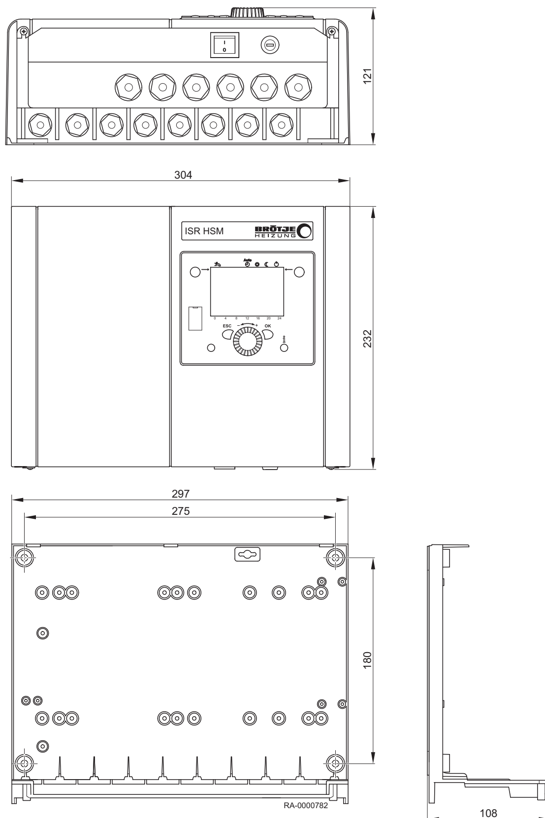
Rys.1 Wymiary
