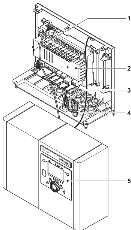
Rys.3 Widok ogólnyHSM
