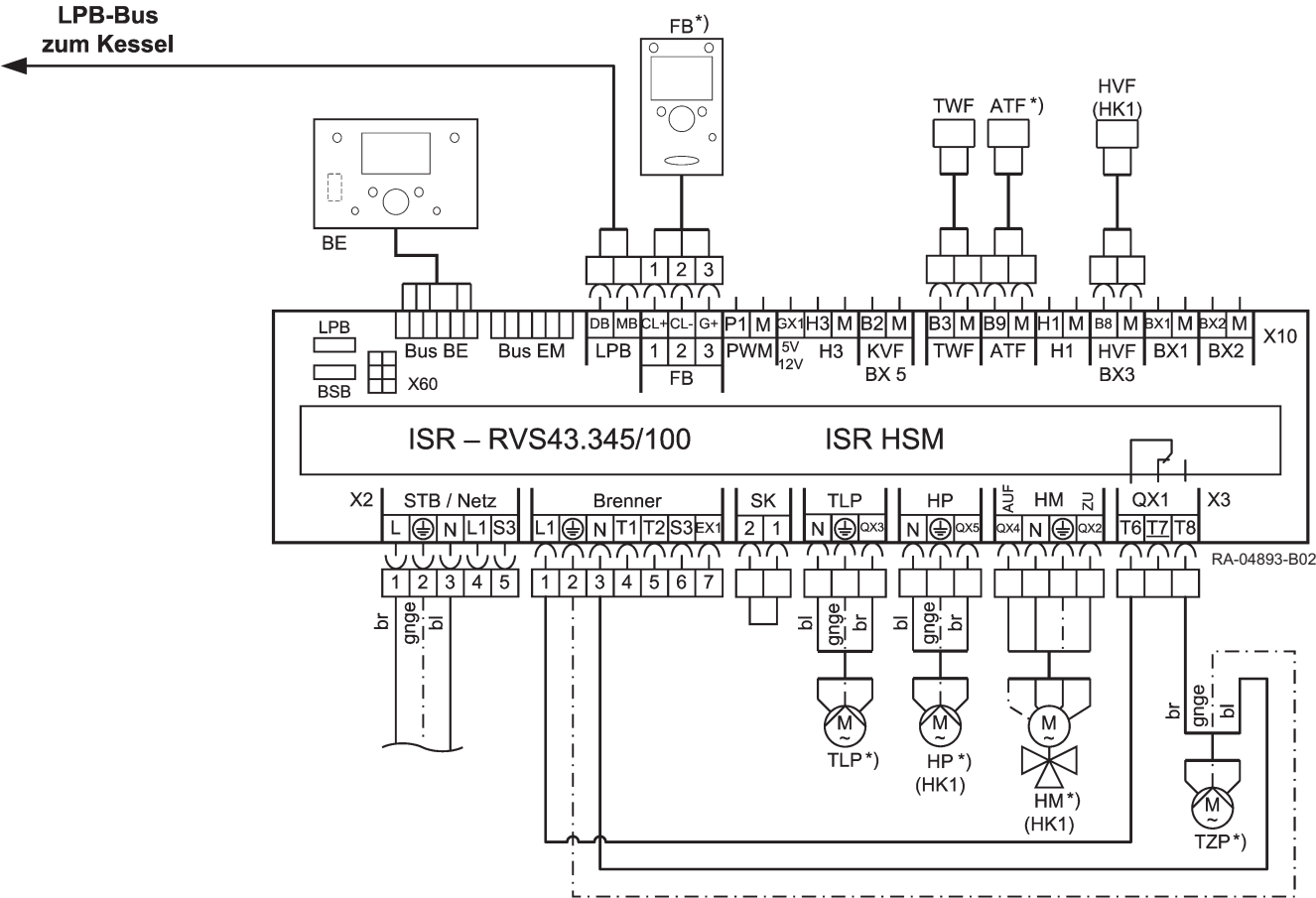
Rys.7 Schemat połączeń elektrycznych
