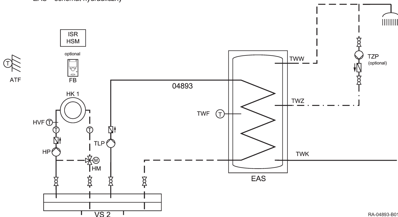
Rys.6 Przykładowa instalacja 1: obieg c.o. z zaworem mieszającym, z regulatorem pokojowym i z podgrzewaczem c.w.u. EAS – schemat hydrauliczny
