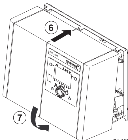
Rys.14 Zamykanie obudowy
