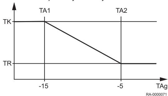
Rys.22 Podwyższanie zredukowanej temperatury zadanej
