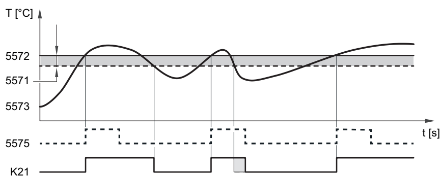
Rys.29 Monitorowanie zbyt wysokiej temperatury
