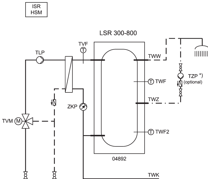
Rys.10 Przykładowa instalacja 3: podgrzewanie c.w.u. w podgrzewaczach c.w.u. LSR 300-800, z regulatorem dodatkowym – schemat hydrauliczny
