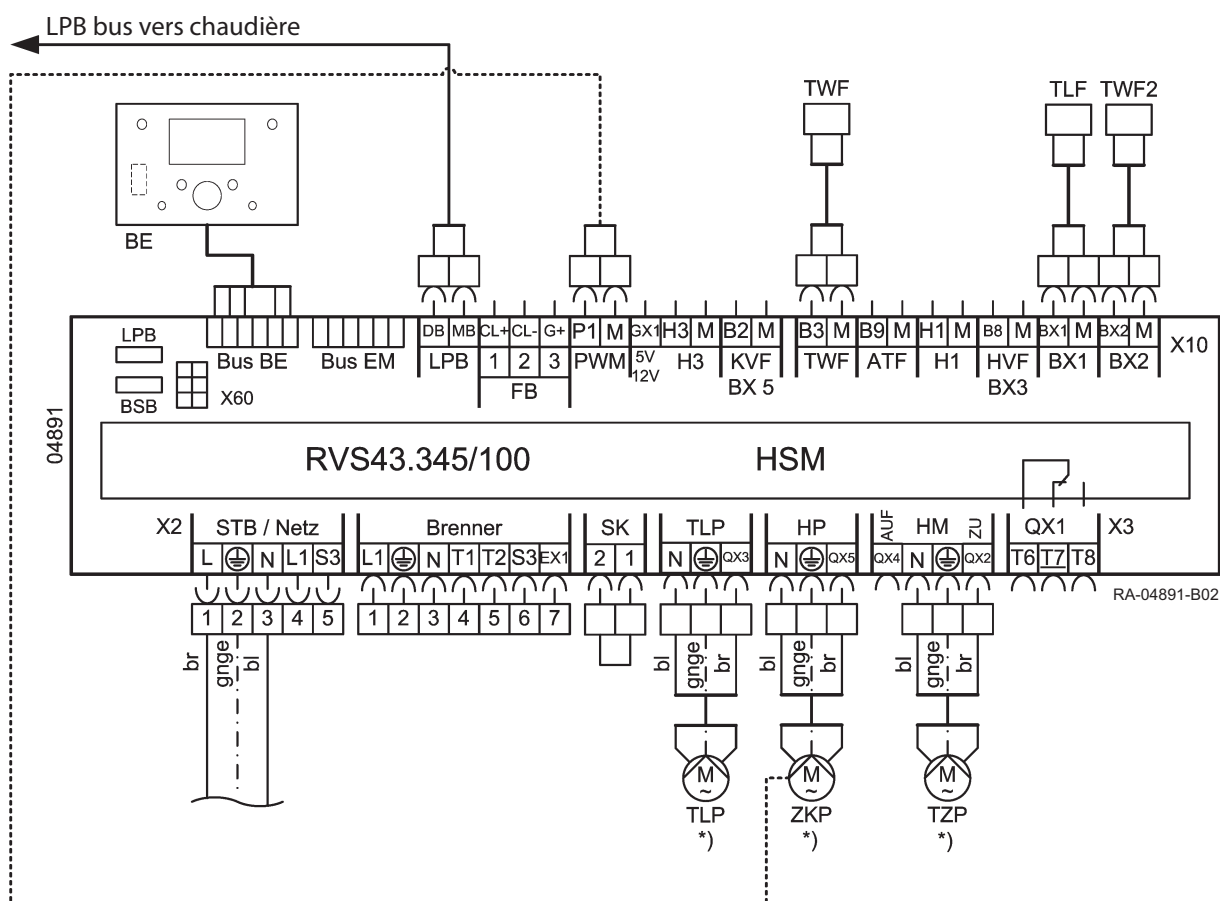
Rys.9 Schemat połączeń elektrycznych
