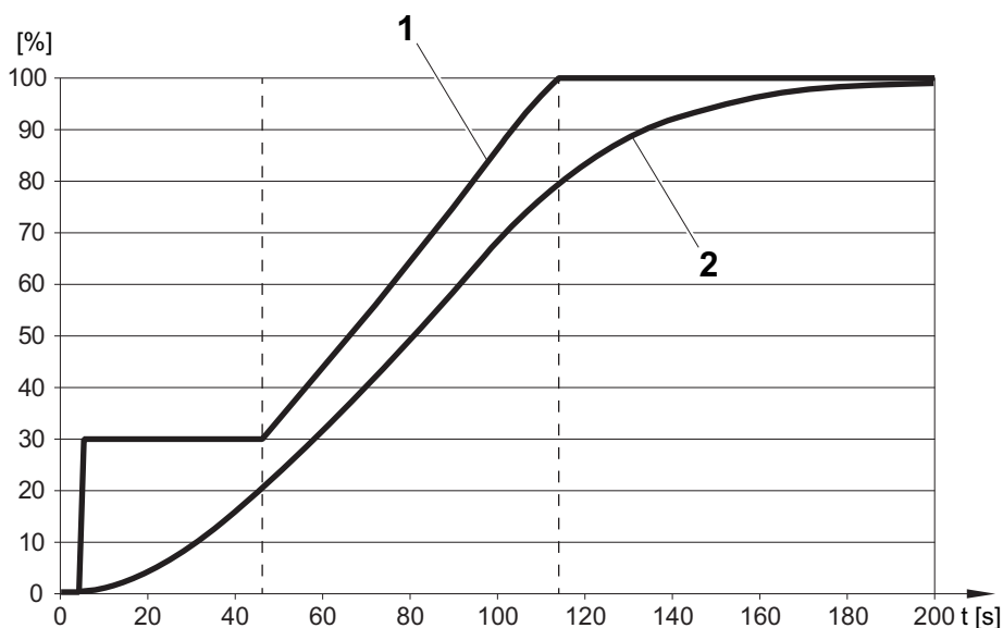
Rys.26 Zależność prędkości obrotowej pompy od mocy źródła ciepła
