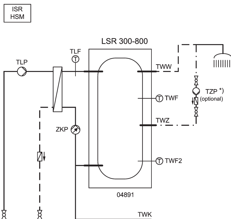
Rys.8 Przykładowa instalacja 2: podgrzewanie c.w.u. w podgrzewaczach c.w.u. LSR 300-800 – schemat hydrauliczny
