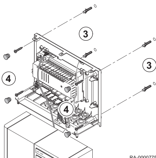
Rys.14 Zamykanie obudowy
