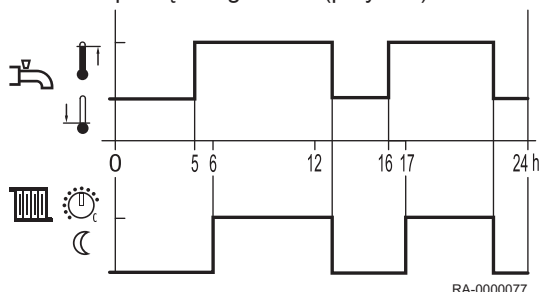
Rys.25 Uruchamianie zgodnie z 4. programem sterowania zegarowego (przykład)
