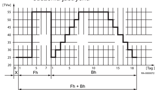
Rys.23 Profil temperaturowy funkcji suszenia jastrychu
