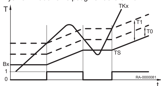
Rys.28 Ładowanie podgrzewacza c.w.u.
