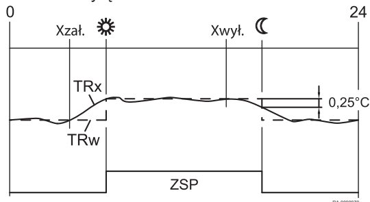
Rys.21 Optymalizacja załączania i wyłączania
