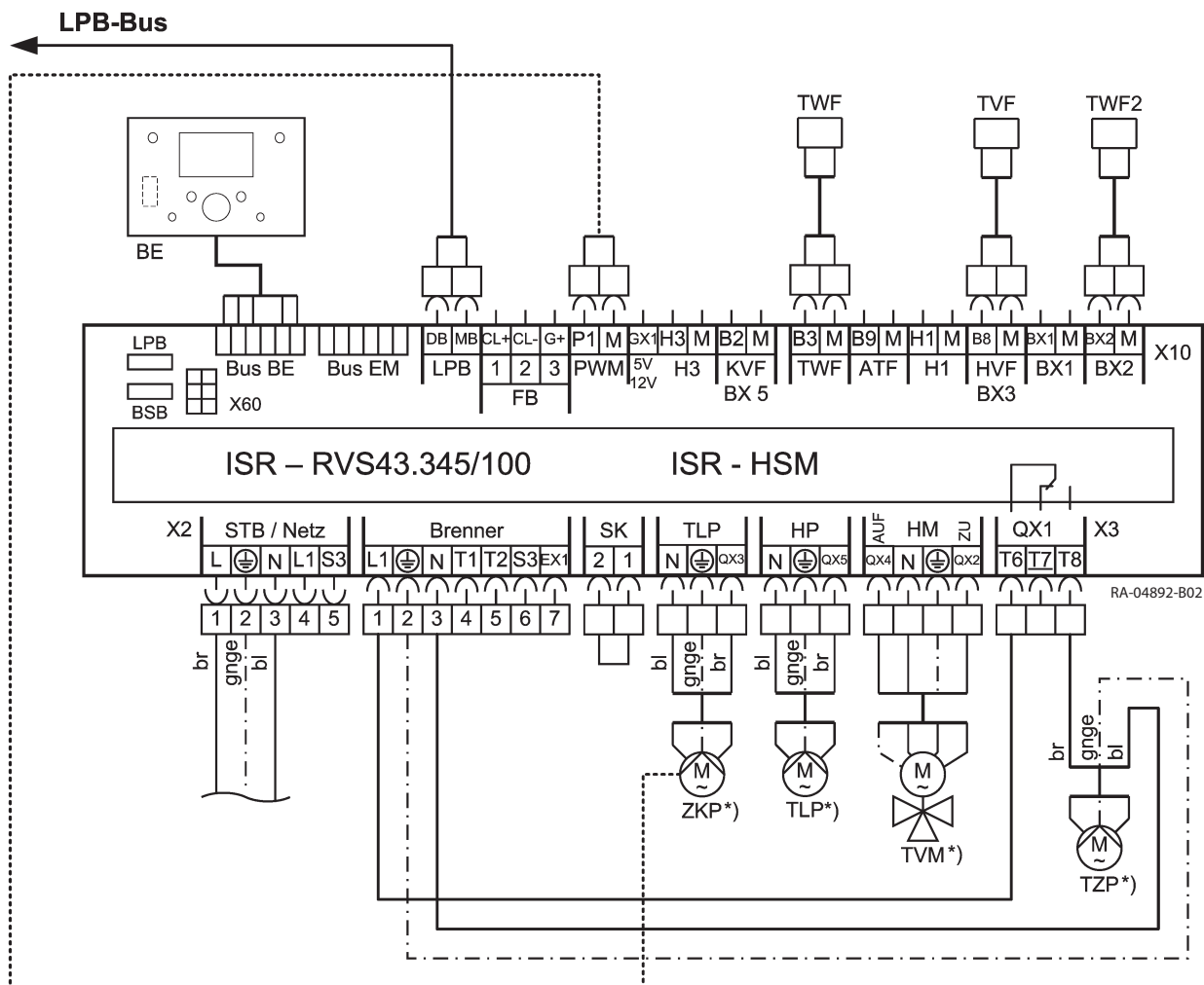
Rys.11 Schemat połączeń elektrycznych
