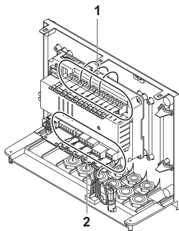
Rys.15 Prowadzenie kabli wewnątrz obudowy
