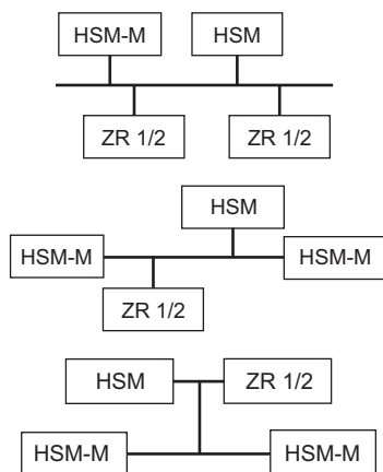
Rys.16 Możliwości podłączenia
