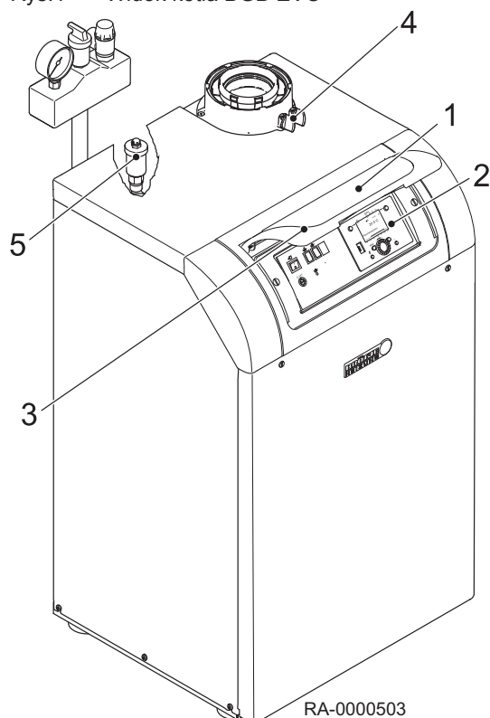
Rys.1 Widok kotła BGB EVO
