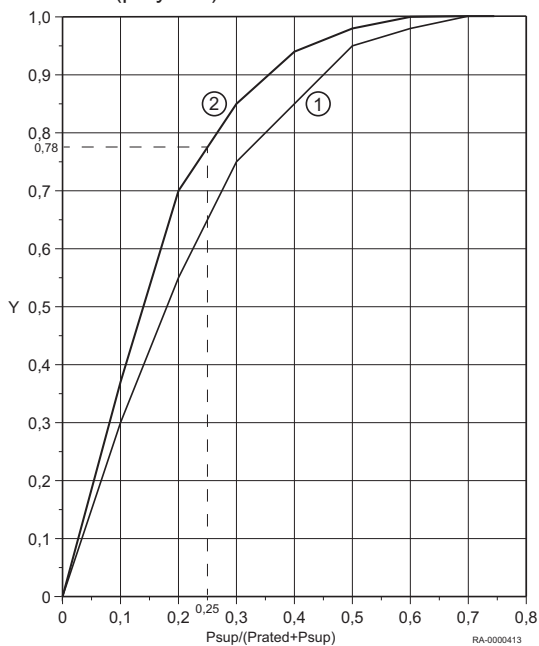
Rys.6 Interpolacja wartości pośrednich (przykład)
