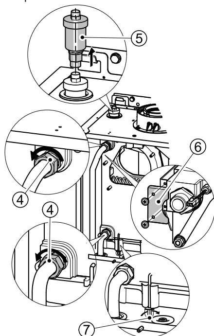
Rys.40 Wymontowywanie wymiennika ciepła
