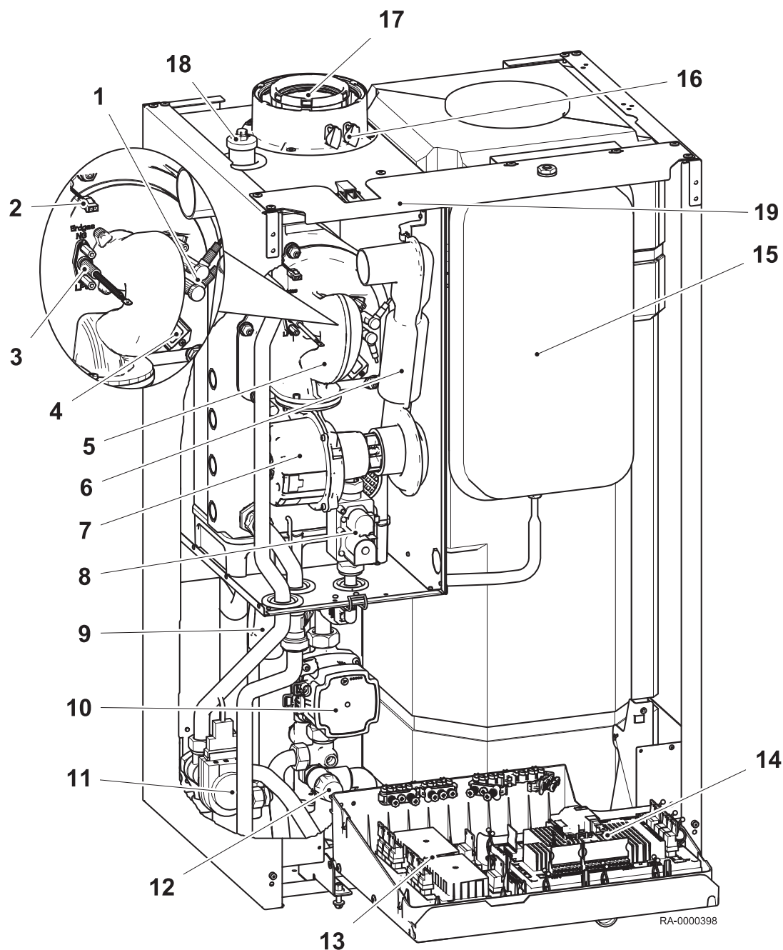
Rys.4 Widok kotła WGB-K EVO (na rysunku bez przedniej ścianki i pokrywy modułu regulacyjnego)
