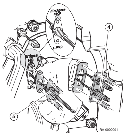
Rys.38 Wymontowywanie elektrody zapłonowej i jonizacyjnej
