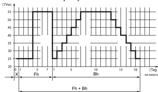
Rys.29 Profil temperaturowy funkcji suszenia jastrychu
