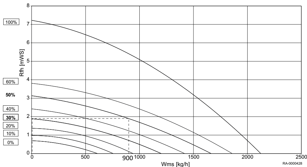
Rys.22 Przykład łącznego ciśnienia dynamicznego
