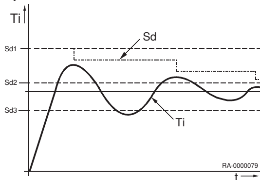
Rys.32 Histereza
