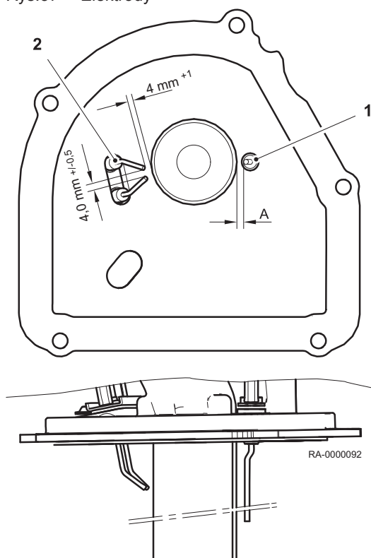
Rys.37 Elektrody
