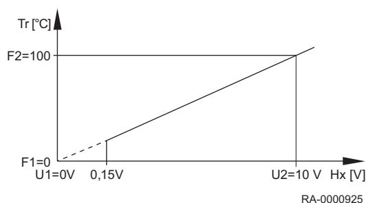
Rys.33 Wartość_napięcia/Wartość_funkcji
