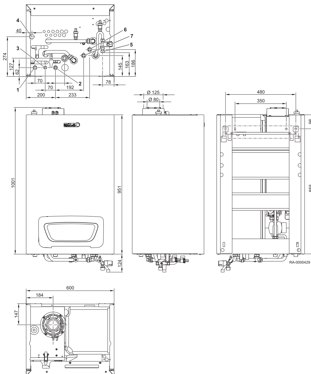
Rys.2 Wymiary i przyłącza kotła WGB-K EVO
