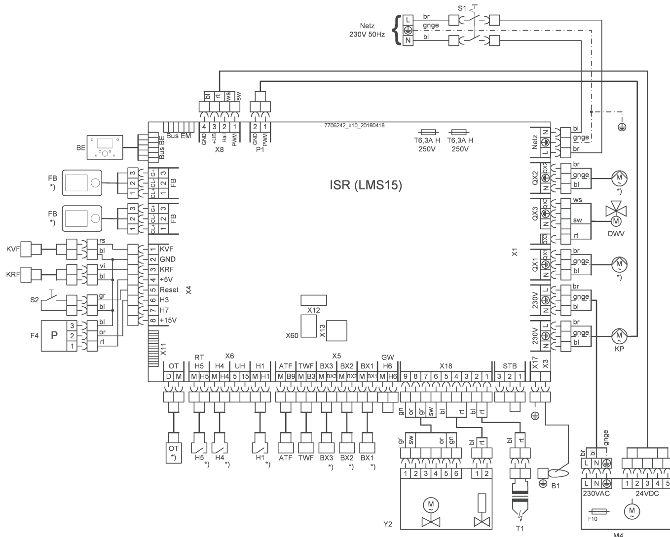
Rys.3 Schemat połączeń elektrycznych kotła WGB-K EVO
