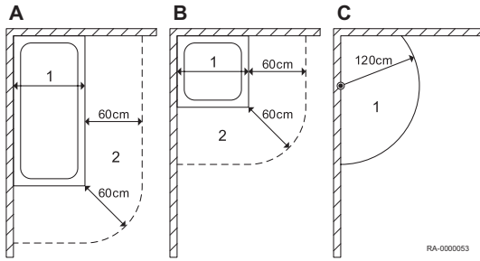
Rys.8 Odległości w łazienkach i pomieszczeniach z prysznicami
