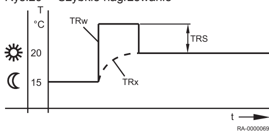
Rys.29 Szybkie nagrzewanie
