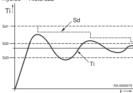
Rys.35 Histereza
