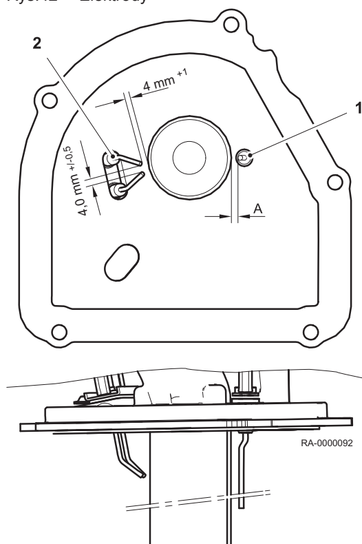
Rys.42 Elektrody
