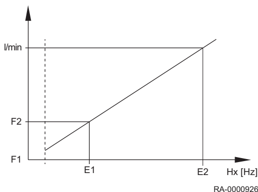
Rys.39 Przykład dwóch różnych charakterystyk czujnika
