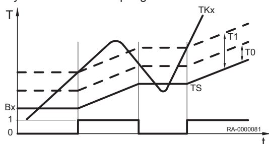
Rys.37 Ładowanie podgrzewacza
