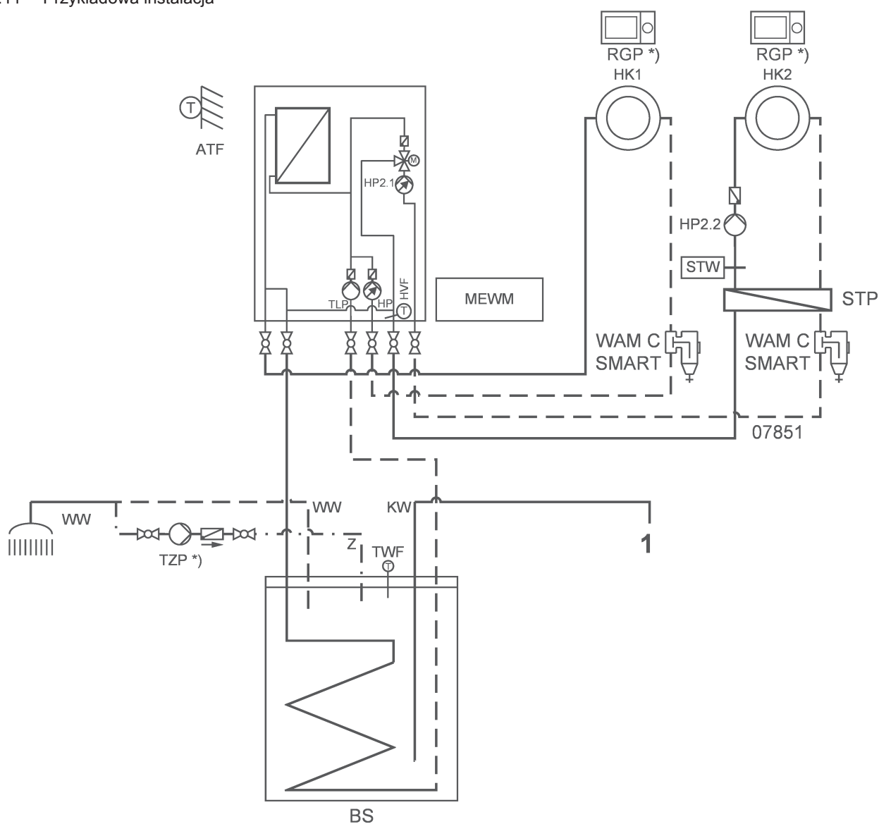
Rys.11 Przykładowa instalacja
