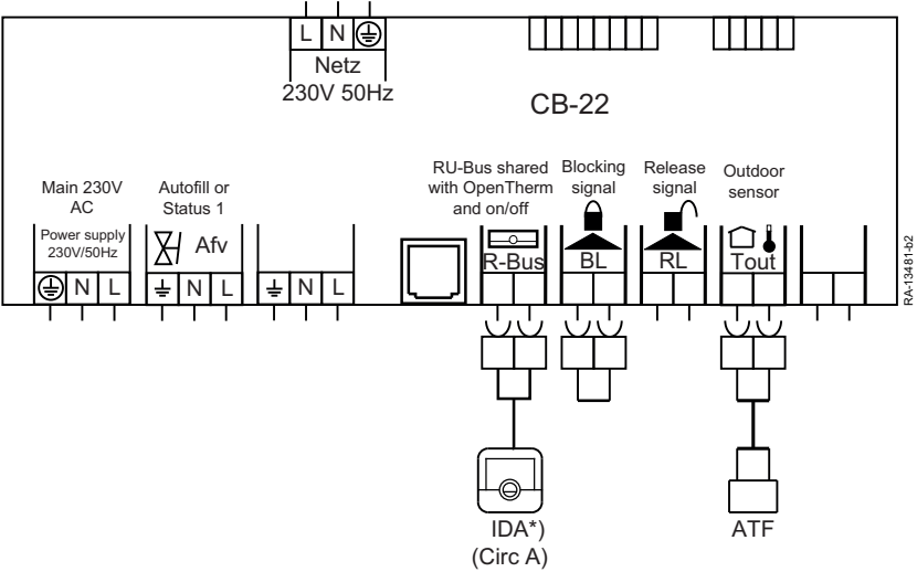
Rys. 15 Schemat połączeń elektrycznych
