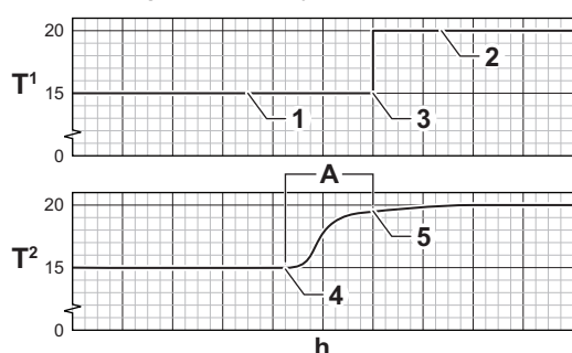
Rys. 58 Wyprzedzające podwyższanie temperatury w pomieszczeniach a program czasowy
