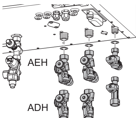
Rys. 17 Montaż zaworów odcinających
