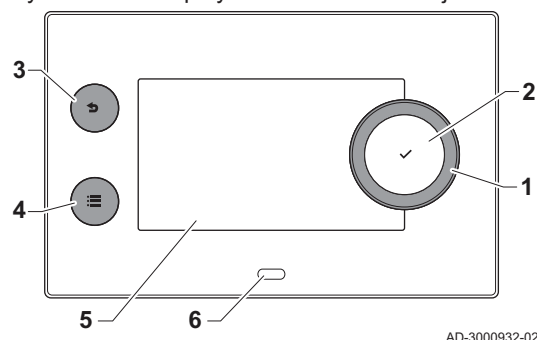
Rys. 7 Podzespoły konsoli sterowniczej
