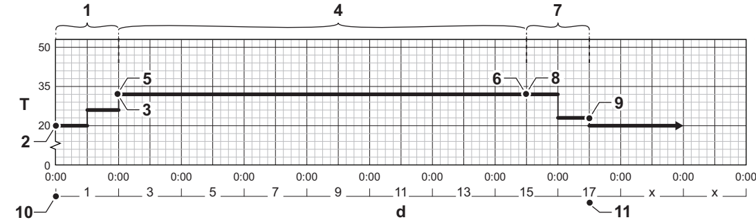
Rys. 55 Charakterystyka osuszania posadzki
