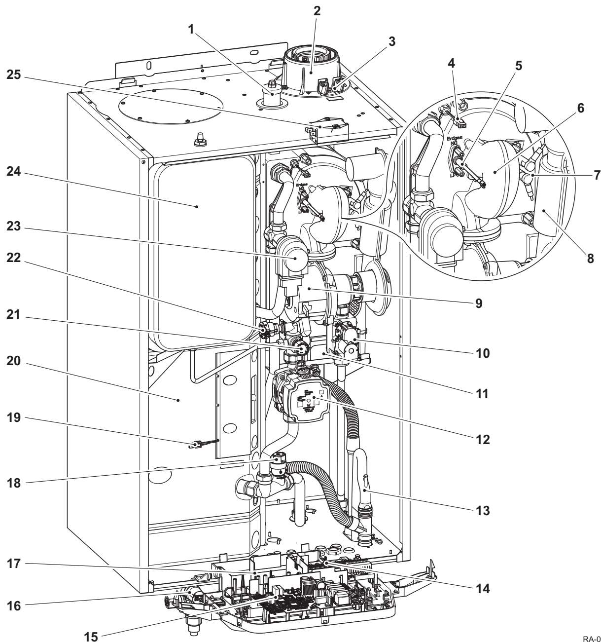
Rys. 6 Widok kotła WGB-K (na rysunku bez przedniej obudowy i pokrywy regulatora)
