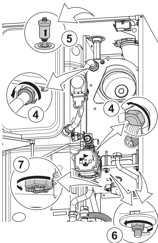
Rys. 70 Wymontowywanie wymiennika ciepła (przygotowanie)
