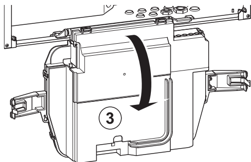
Rys. 64 Wychylanie regulatora kotła całkowicie do dołu.
