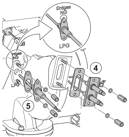
Rys. 67 Wymontowywanie elektrody zapłonowej i jonizacyjnej
