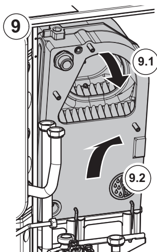
Rys. 71 Wymontowywanie wymiennika ciepła
