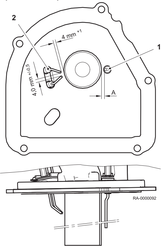
Rys. 66 Elektrody
