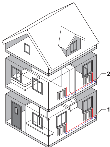
Rys. 10 Dwa obiegi grzewcze (c.o.)
