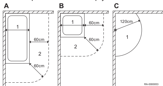
Rys. 13 Odległości w łazienkach i pomieszczeniach z prysznicami
