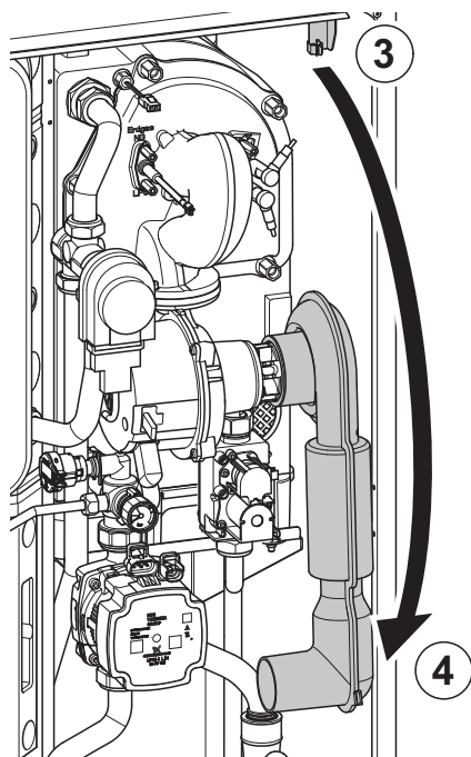
Rys. 69 Wymontowywanie palnika gazowego
