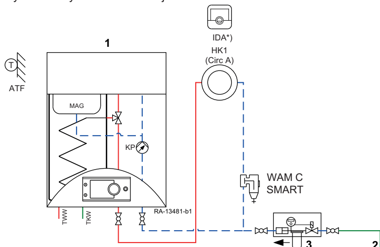
Rys. 14 Przykładowa instalacja
