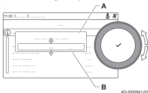
Rys. 36 Test niskiego obciążenia
