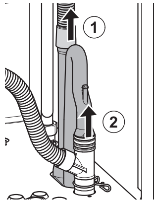
Rys. 65 Wymontowywanie syfonu
