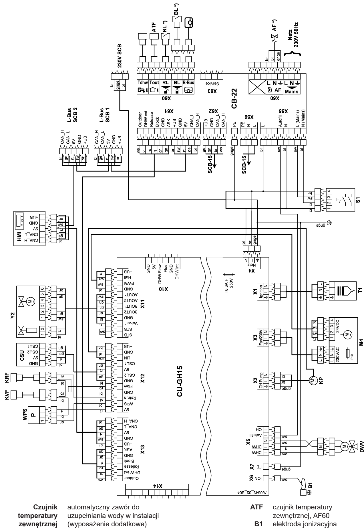
Rys. 4 Schemat połączeń elektrycznych kotłów CU-GH15 WGB-K 22/28.1
