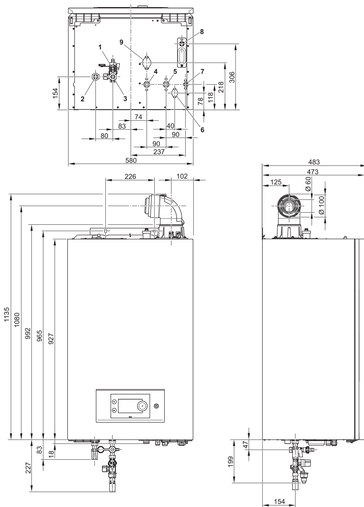
Rys. 2 Wymiary kotłów WGB-K 22/28.1
