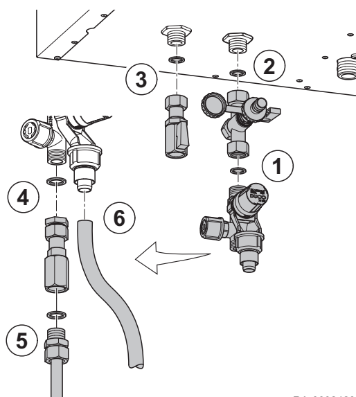
Rys. 16 Montowanie grupy bezpieczeństwa c.w.u.
