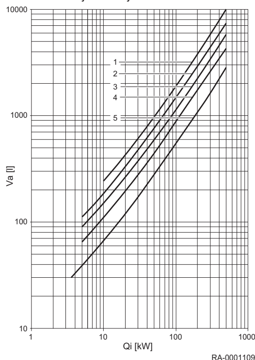
Rys. 12 Określanie szacunkowej pojemności wodnej instalacji
