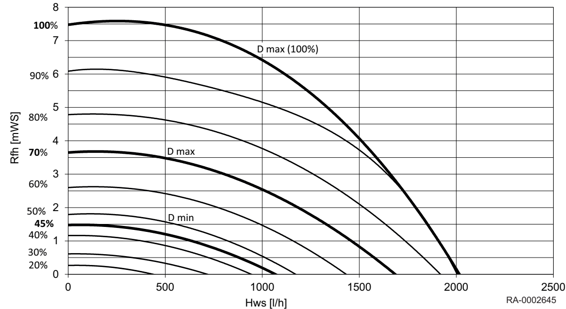
Rys. 1 Dyspozycyjna wysokość podnoszenia WGB-K 22/28.1
