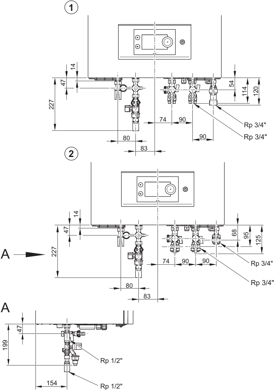
Rys. 3 Wymiary kotłów WGB-K z zestawami zaworów odcinających AEH B/ADH B
