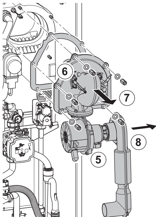
Rys. 69 Wymontowywanie palnika gazowego
