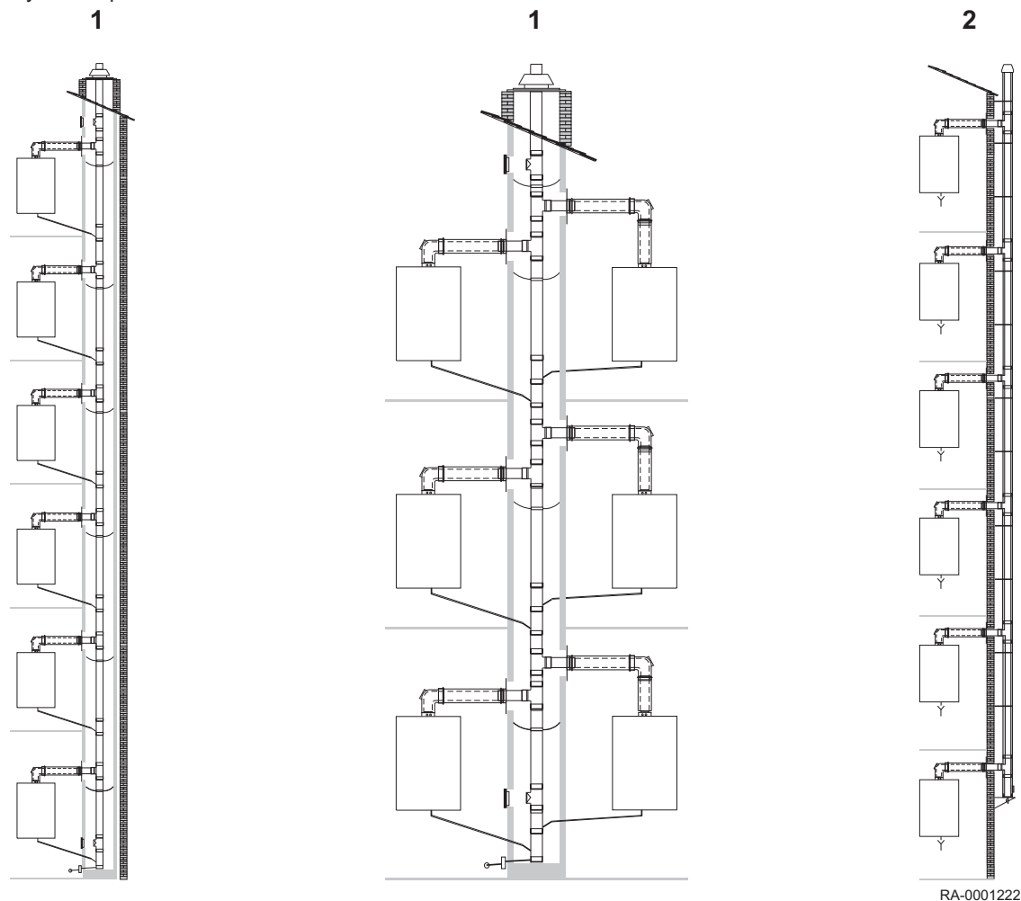
Rys. 23 Sposób montażu
