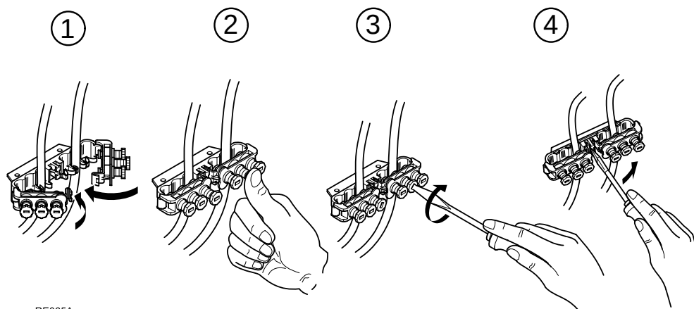
Rys. 9: Dławik przewodu
