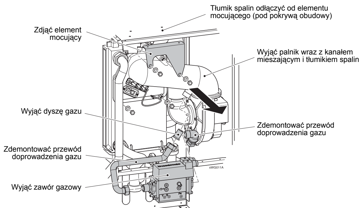
Rys. 21: Wymontować palnik gazowy (kocioł WGB 70 C)
