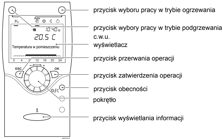
Rys. 19: Panel obsługowy regulatorów RGT
