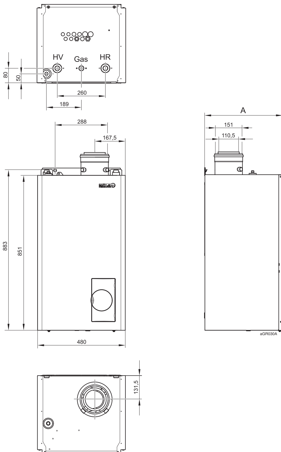
Rys. 1: Wymiary i przyłącza
