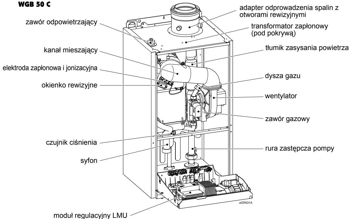
Rys. 22: Widok kotła (na rysunku bez przedniej ścianki obudowy i pokrywy zespołu regulacyjnego)
