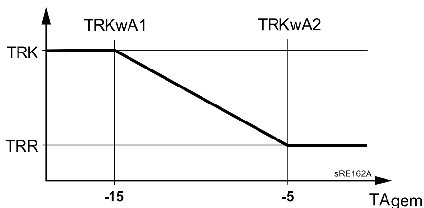
Rys. 20: Zred. obniż.
