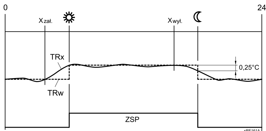
Rys. 19: Optymalizacja załączania i wyłączania
