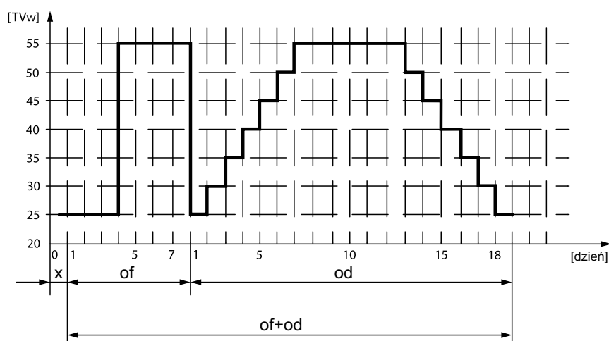
Rys. 21: Profil temperatury dla funkcji osuszania jastrychu
