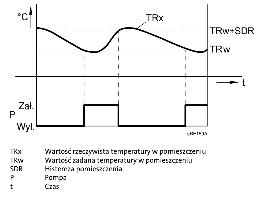
Rys. 17: Ograniczenie temp. w pom.
