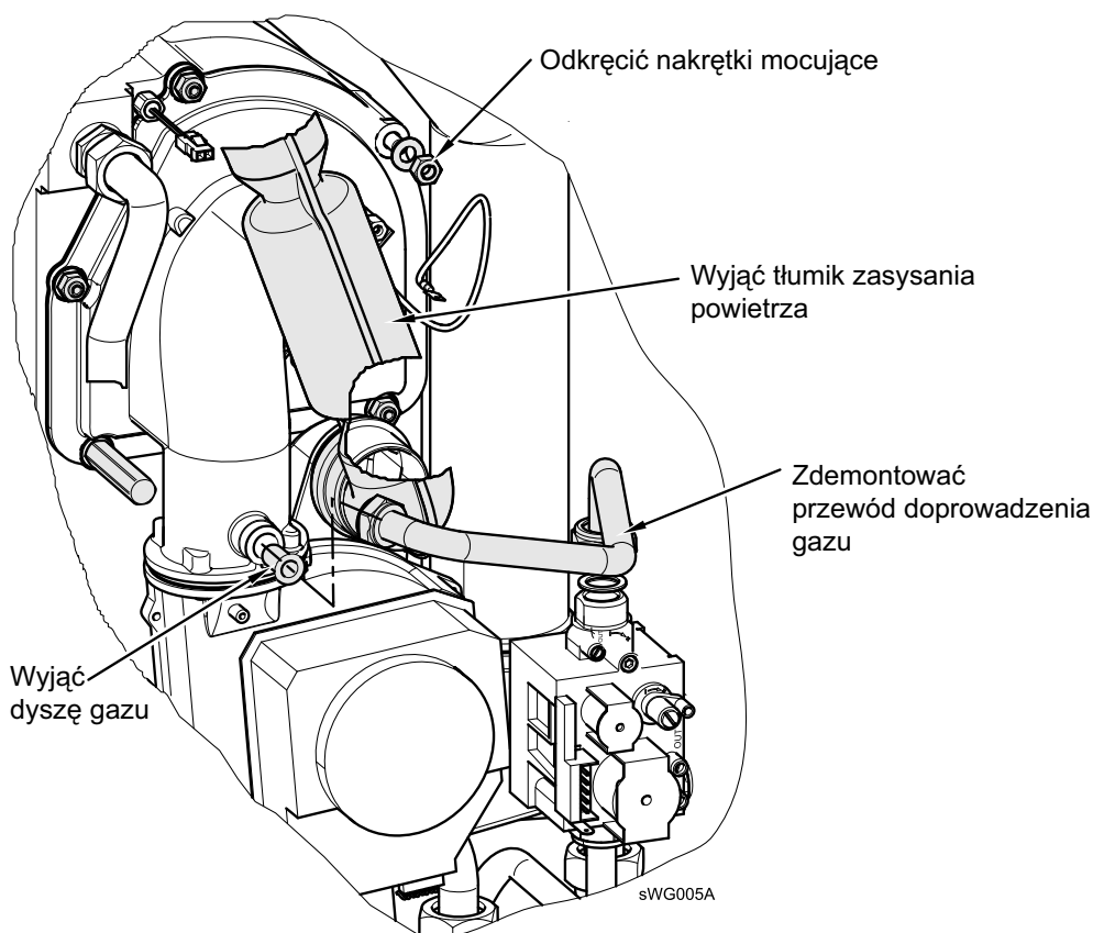
Rys. 27: Wymontowywanie palnika gazowego
