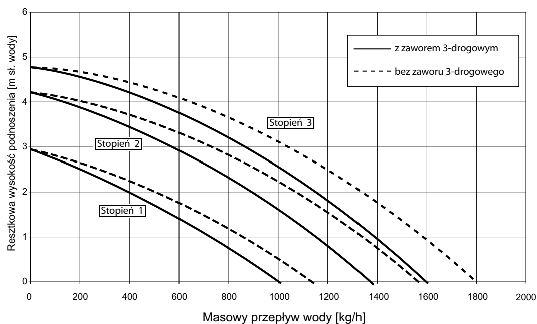
Rys. 22: Resztkowa wysokość podnoszenia WBC 22/24 E
