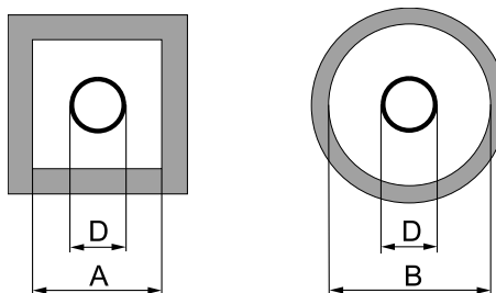
Rys. 10: Minimalne wymiary przewodu kominowego
