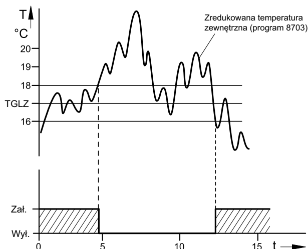
Rys. 16: Temp. graniczna lato/zima
