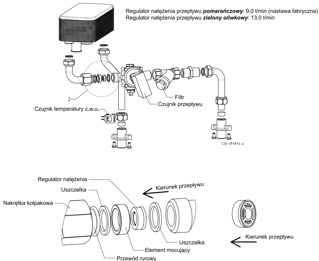
Rys. 6: Wymiana regulatora przepływu
