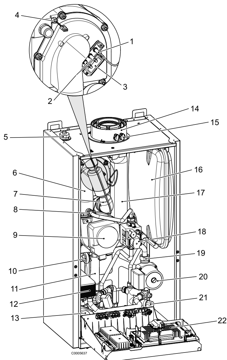
Rys. 28: Widok kotła WBC (na rysunku bez przedniej ścianki i pokrywy modułu regulacyjnego)
