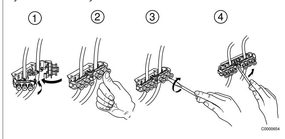
Rys. 12: Dławik kablowy
