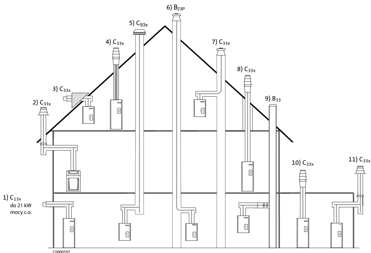
Rys. 7: Możliwości zamontowania kotła z zastosowaniem systemu KAS (wyposażenie dodatkowe)
