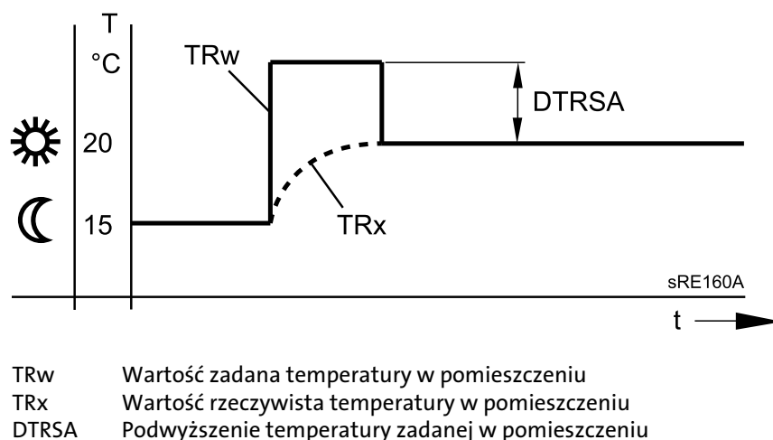
Rys. 18: Szybkie nagrzewanie
