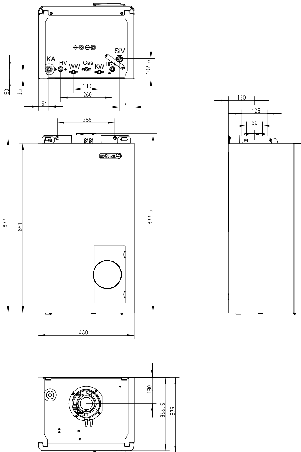
Rys. 1: Wymiary i przyłącza kotła
