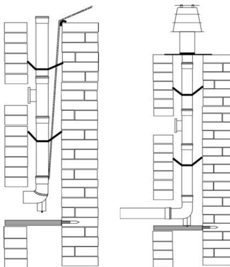
Rys. 9: Wprowadzanie przewodu odprowadzenia spalin do przewodu kominowego
