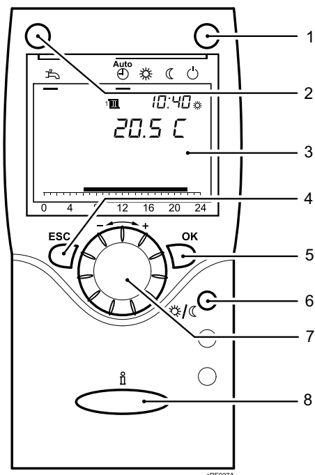
Rys. 26: Panel obsługi regulatorów RGT
