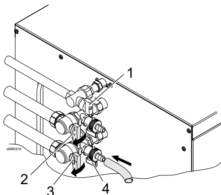
Rys. 5: Zamknąć zawory odcinające i zawór odcinający dopływ gazu
