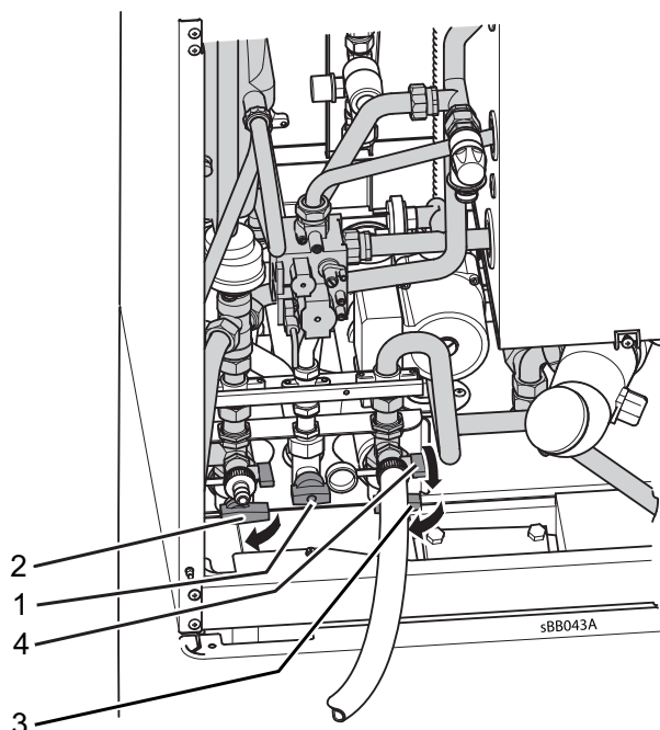
Rys. 6: Zamknąć zawory odcinające i zawór odcinający dopływ gazu
