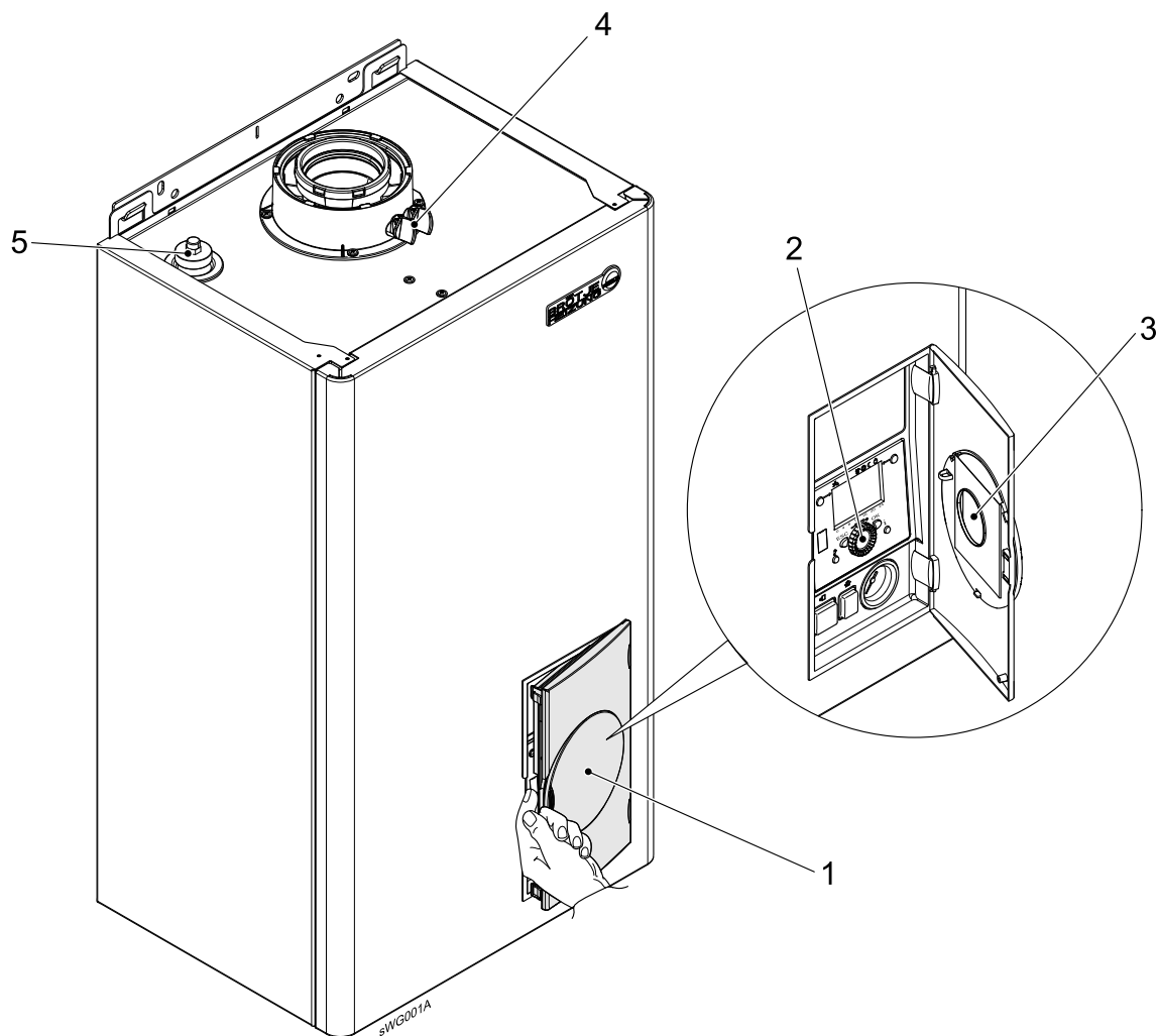
Rys. 1: Rysunek poglądowy kotła WBS / WBC
