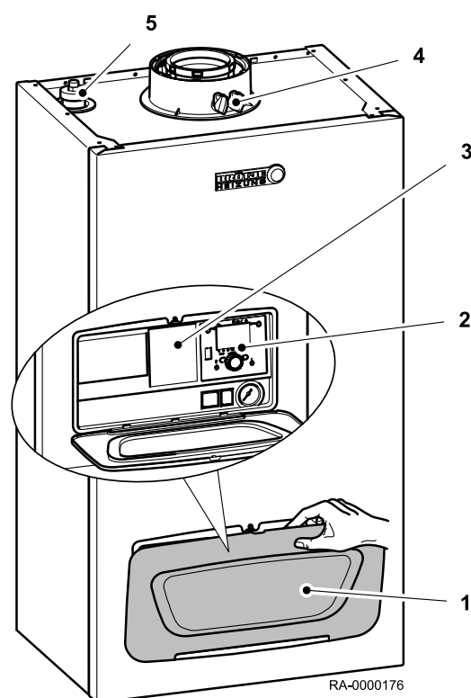
Rys.1 Widok kotła WBC/WBS
